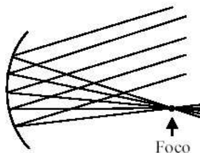
Figura 1.1: Raios paralelos entre si incidem em um espelho côncavo e refletem sobre o foco.
